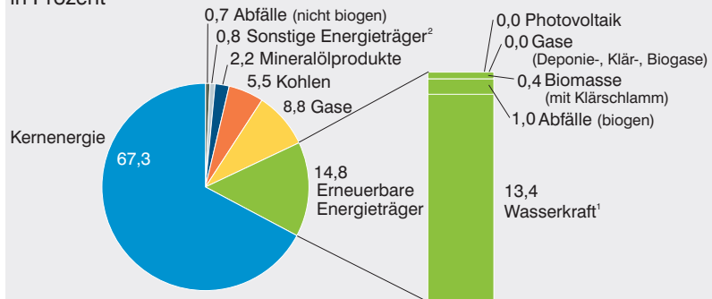
Bruttostromerzeugung in Stromerzeugungsanlagen der allgemeinen Versorgung nach Energieträgern in Bayern 2009 in Prozent
