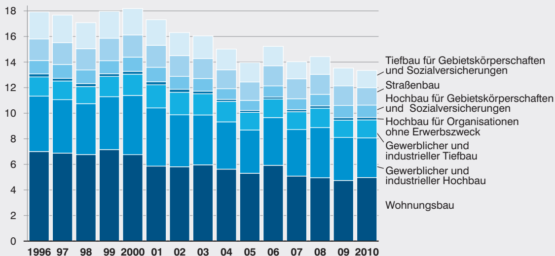
Bauhauptgewerbe in Bayern von 1996 bis 2010 Umsatz nach Bauarten bzw. Arten von Auftraggebern* in Milliarden Euro
