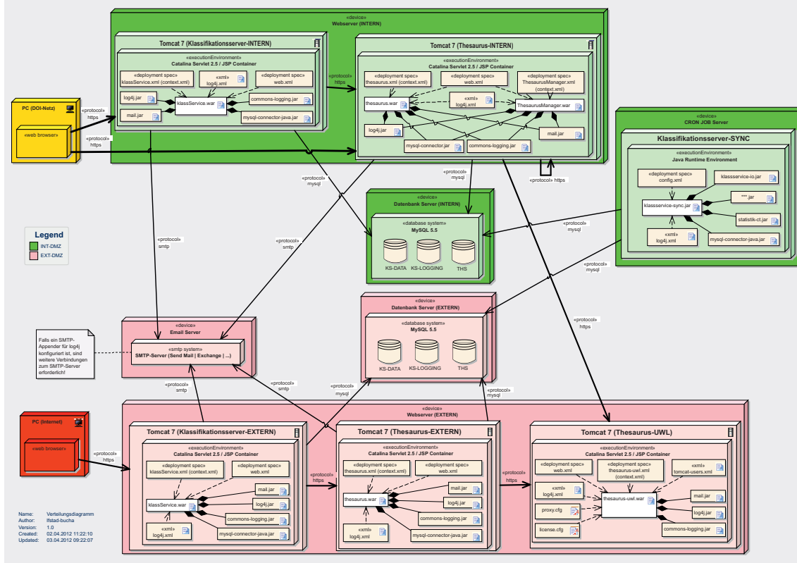
Deployment Verteilungsdiagramm
