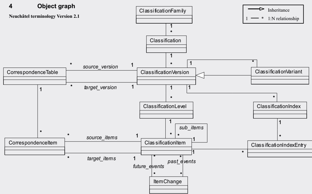
Neuchâtel Modell Objektgraph
