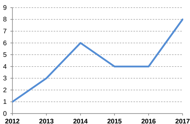
Straßenverkehrsunfälle
