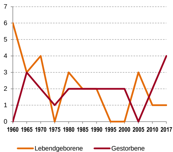
Natürliche Bevölkerungsbewegung
