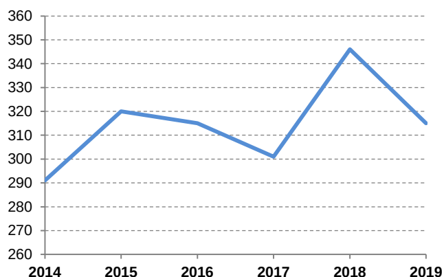
Straßenverkehrsunfälle
