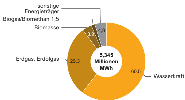
Nettostromerzeugung im 2. Quartal 2024 nach Energieträgern in Prozent
