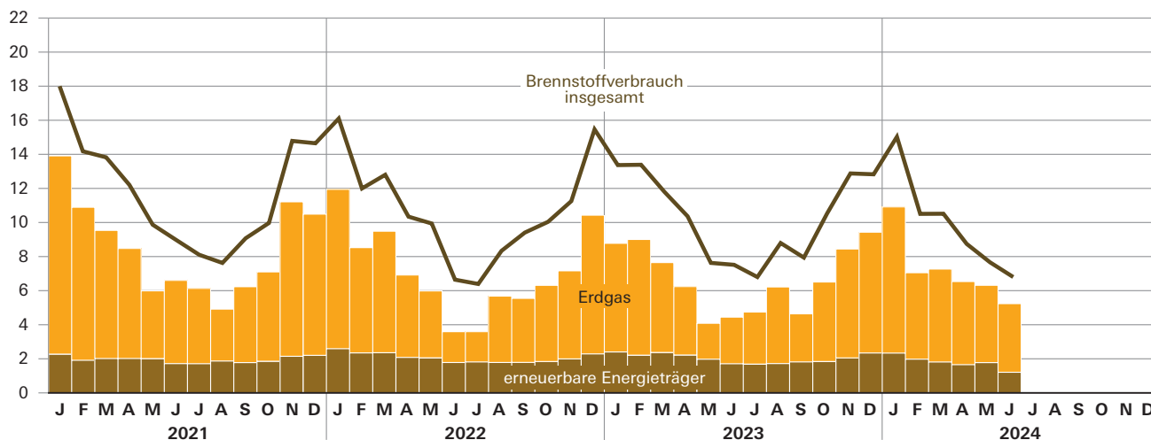
Brennstoffverbrauch in den Jahren 2021 bis 2024 in Millionen Gigajoule (GJ)
