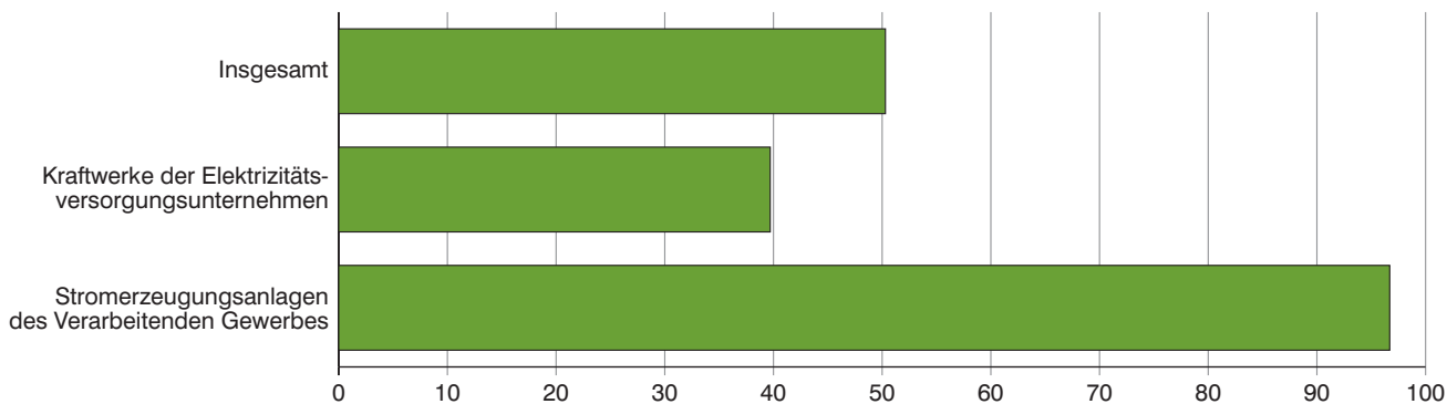
Abb. 5 Anteil Kraft-Wärme-Kopplung bei der Nettostromerzeugung* 2012 nach Anlagenart 5 in Prozent
